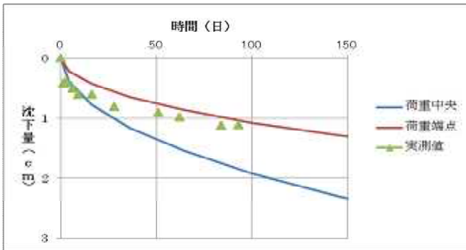
図-4 沈下量と経過日数の関係(岡山浦安)
