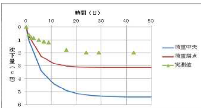
図-5 沈下量と経過日数の関係(諏訪)
