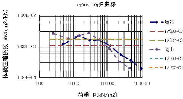
図-3 mvの換算値との比較
