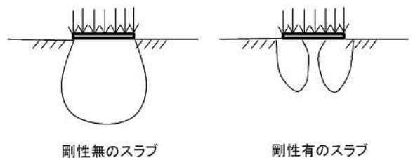
図-6 地中応力の違い
